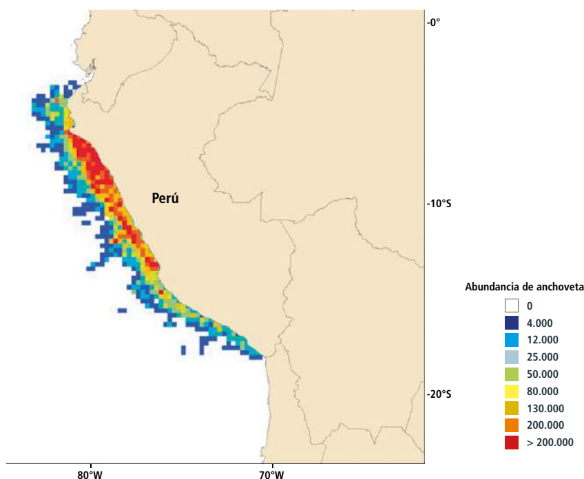
MAPA V.2 Abundancia promedio anual estimada de la anchoveta en la costa peruana, 1983-2006 (En toneladas)
