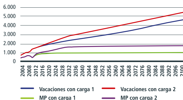
GRÁFICO V.25 Proyección de turistas de vacaciones y capacidad de carga a Machu Picchu al año 2100, escenario base (En número de turistas)
