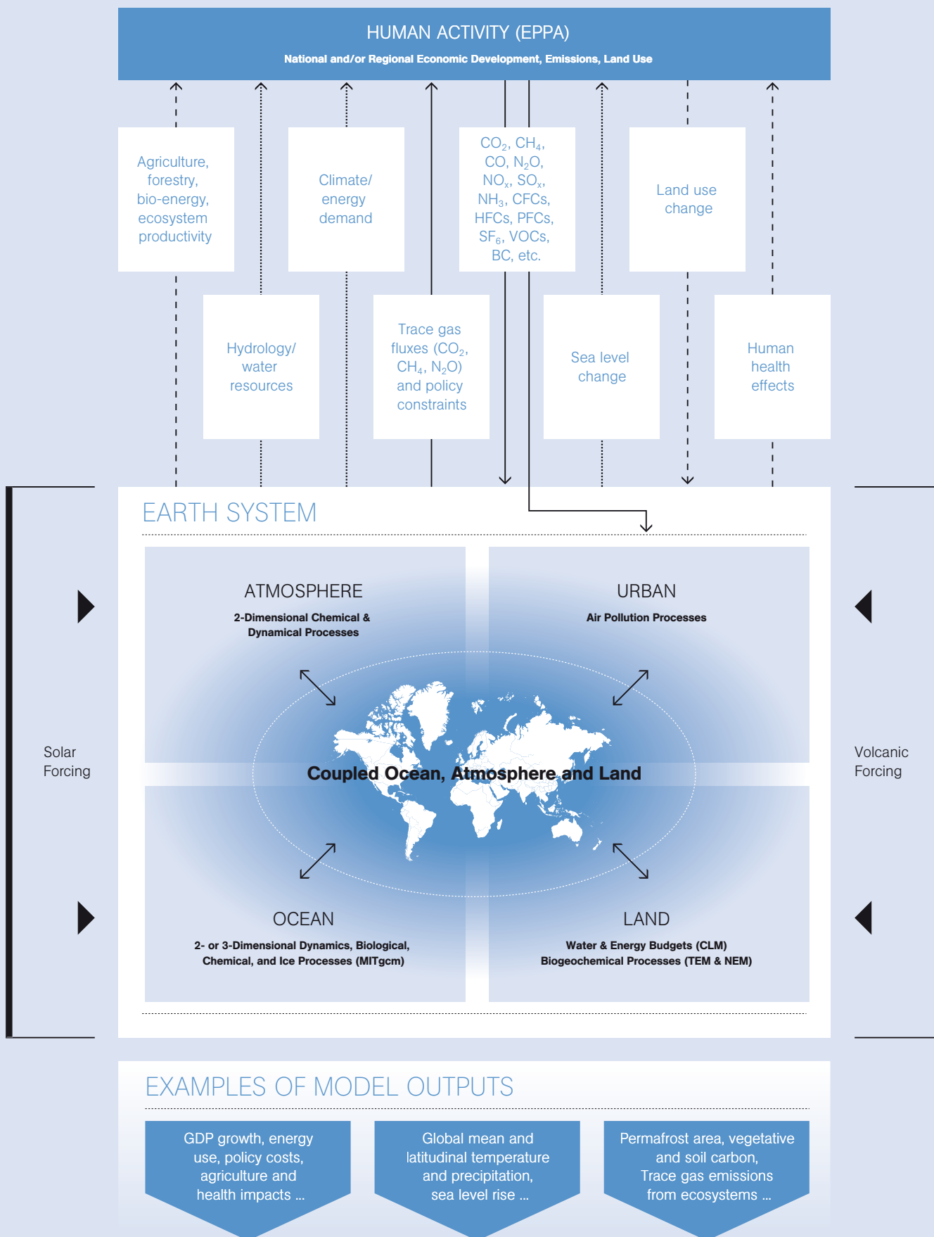
Figure III-4. Schematic of the MIT Integrated Global System Model
