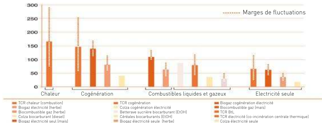
Figura 13: Resumen de producción energética actual (neta) de materias primas renovables por diferentes trayectorias de uso en GJ/ha
