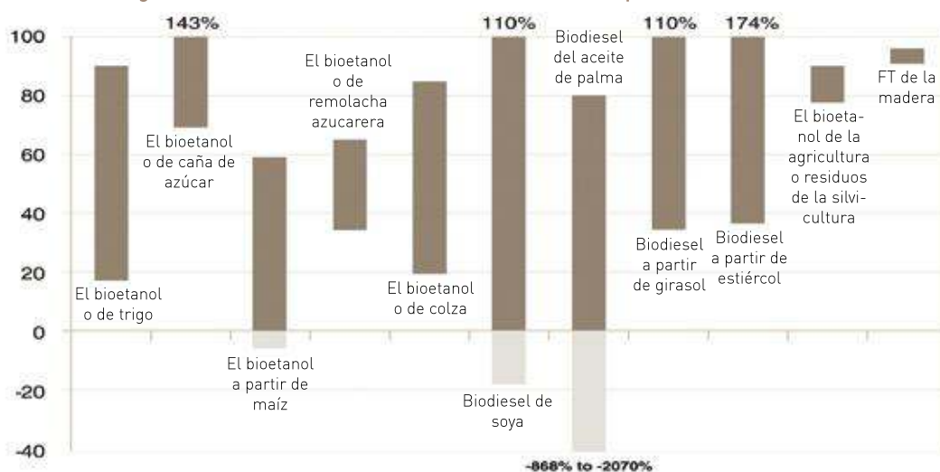
Figura 7: Ahorro de gases de efecto invernadero de biocombustibles en comparación con los combustibles fósiles
