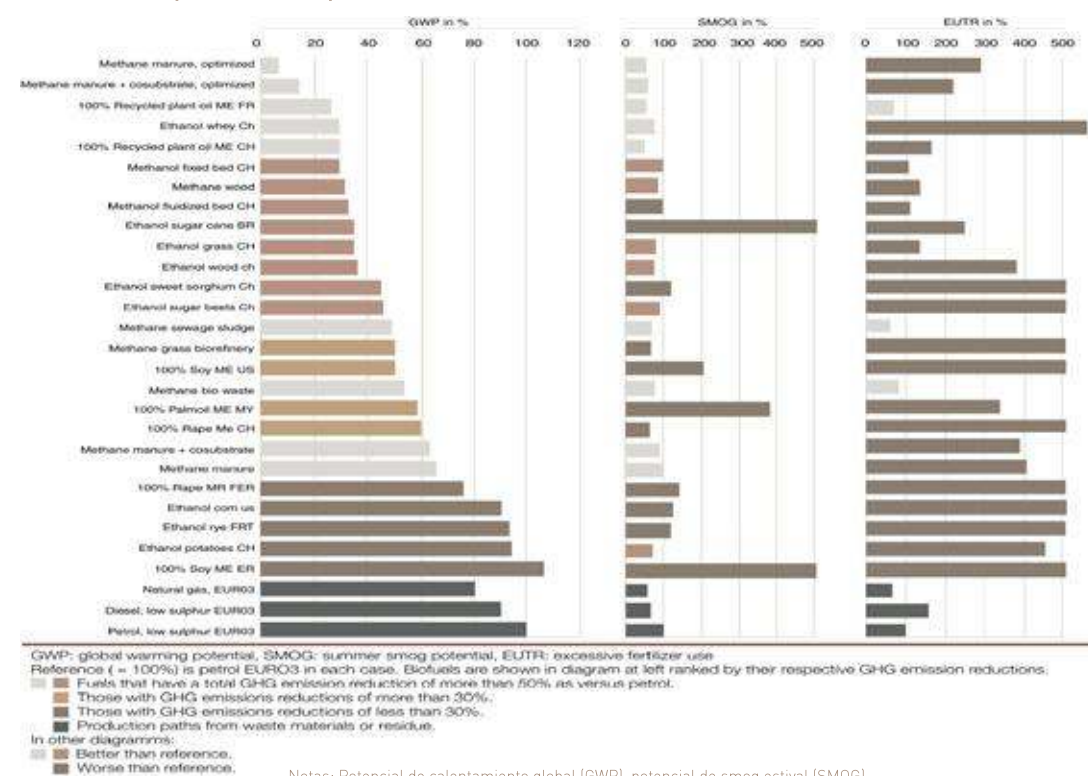
Figura 8: Evaluación del impacto del ciclo de vida de los biocombustibles comparado con los combustibles fósiles para diferentes presiones medioambientales
