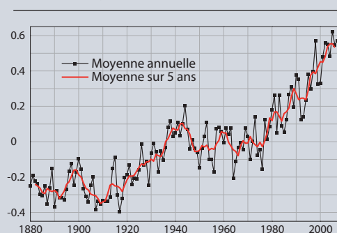
Figure 1 : Changement de la température à la surface
