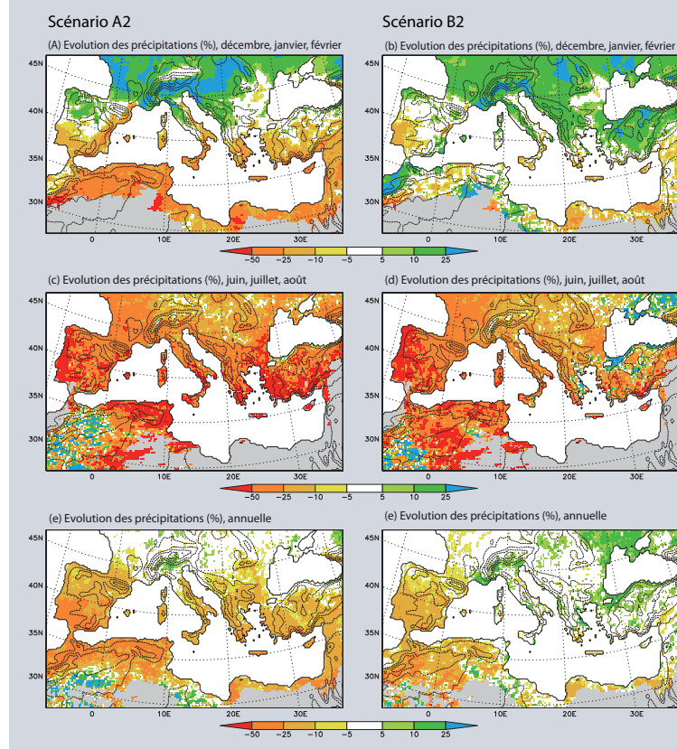
Figure 5 : Deux scénarios pour les changements des précipitations dans la région méditerranéenne
