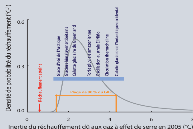
Figure 6 : Distribution des probabilités pour un réchauffement engagé associé à des émissions de gaz à effet de serre entre 1750 et 2005
