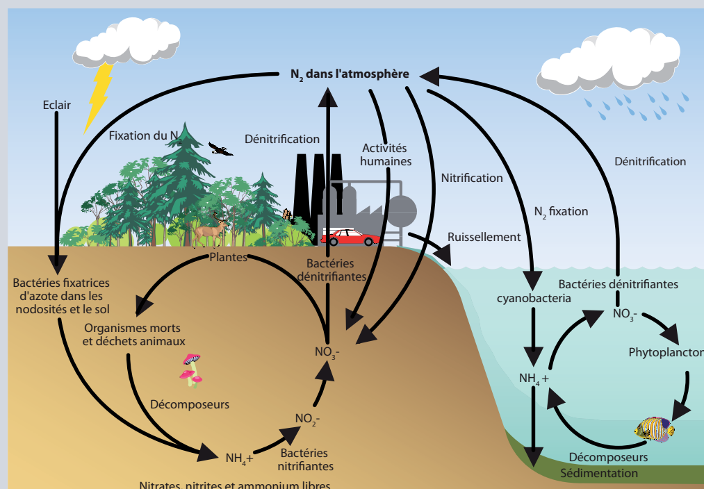
Figure 3 : Cycle de l'azote
