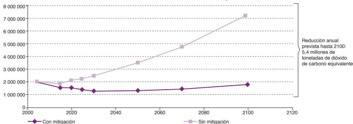
GRÁFICO VI.6 ESCENARIOS PROYECTADOS: EMISIONES DE GASES DE EFECTO INVERNADERO DEL SECTOR RESIDUOS, 2006-2100 (En toneladas de dióxido de carbono equivalente)
