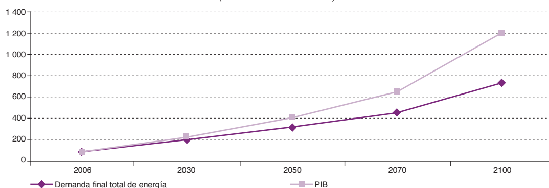
GRÁFICO VI.1 ESCENARIO TENDENCIAL: DEMANDA FINAL TOTAL DE ENERGÍA, 2006-2100 (Año base 2006=100)
