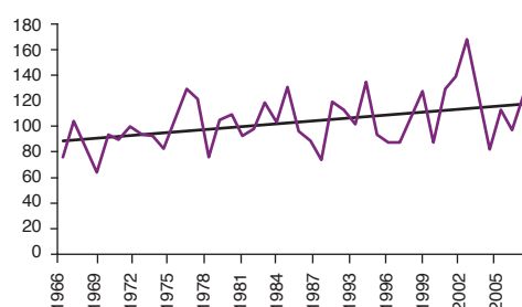
B. Precipitaciones (crecimiento anual: 0,7%), 1966-2006 (En milímetros por mes)
