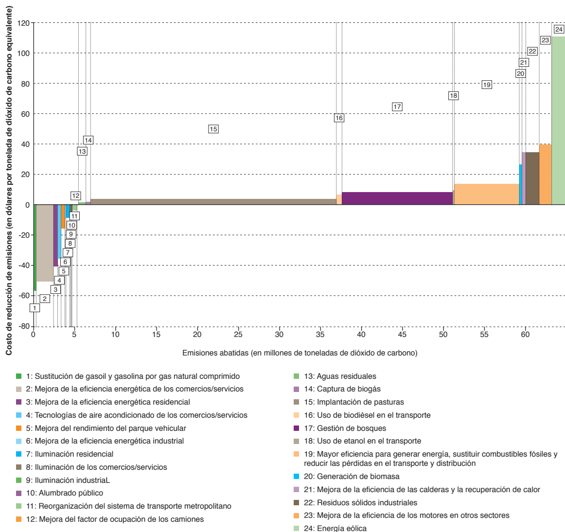
GRÁFICO VI.7 CURVA DE COSTOS DE ABATIMIENTO DE LAS EMISIONES DE GASES DE EFECTO INVERNADERO HASTA 2030
