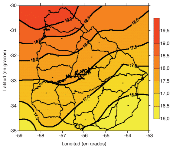
C. Temperatura media anual, 1961-1990 (En grados Celsius)
