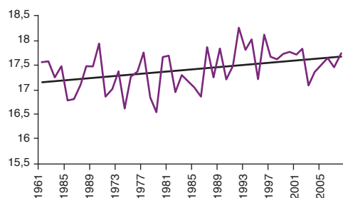
A. Temperatura (crecimiento anual: 0,08%), 1961-2005 (En grados Celsius)
