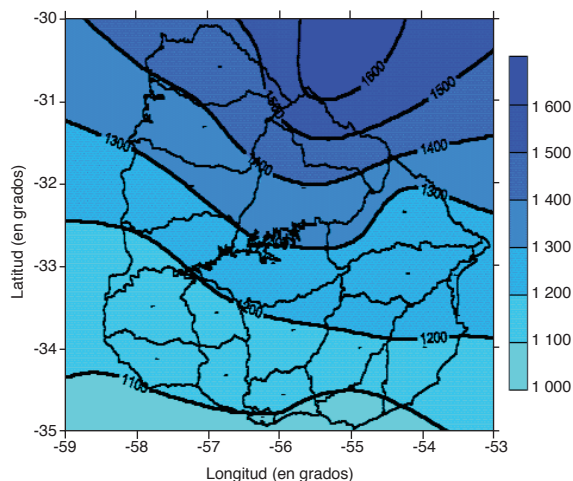
D. Precipitación medial anual, 1961-1990 (En milímetros)
