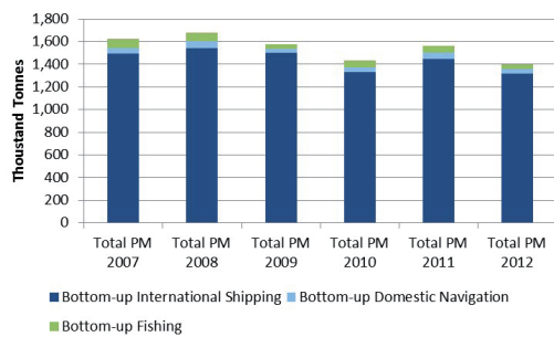
f) PM
