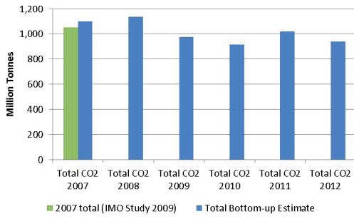
a) CO 2
