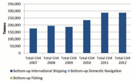
b) CH 4
