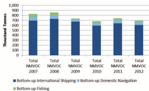
h) NMVOC
