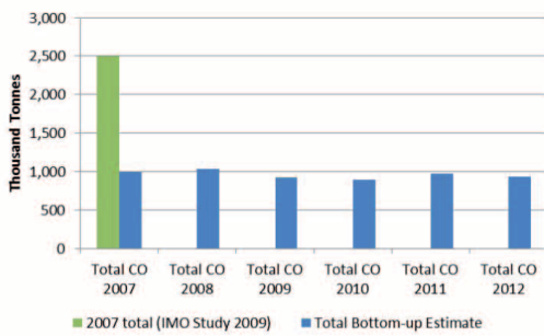
g) CO
