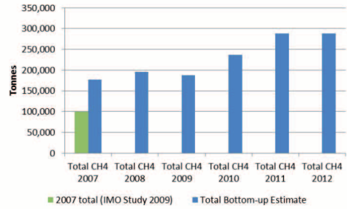
b) CH 4
