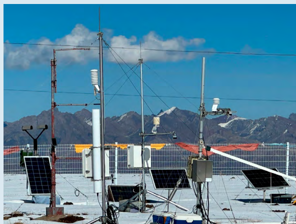
Esempio di stazione idrometeorologica automatizzata INARCH installata in un bacino di alta montagna: Monti Qilian, Cina
