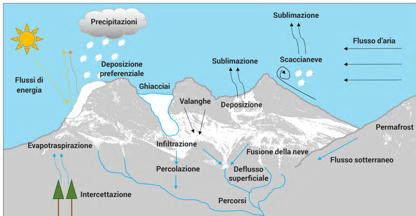
Figura 2.1 Processi idrologici e della criosfera di alta montagna che regolano l'approvvigionamento idrico
