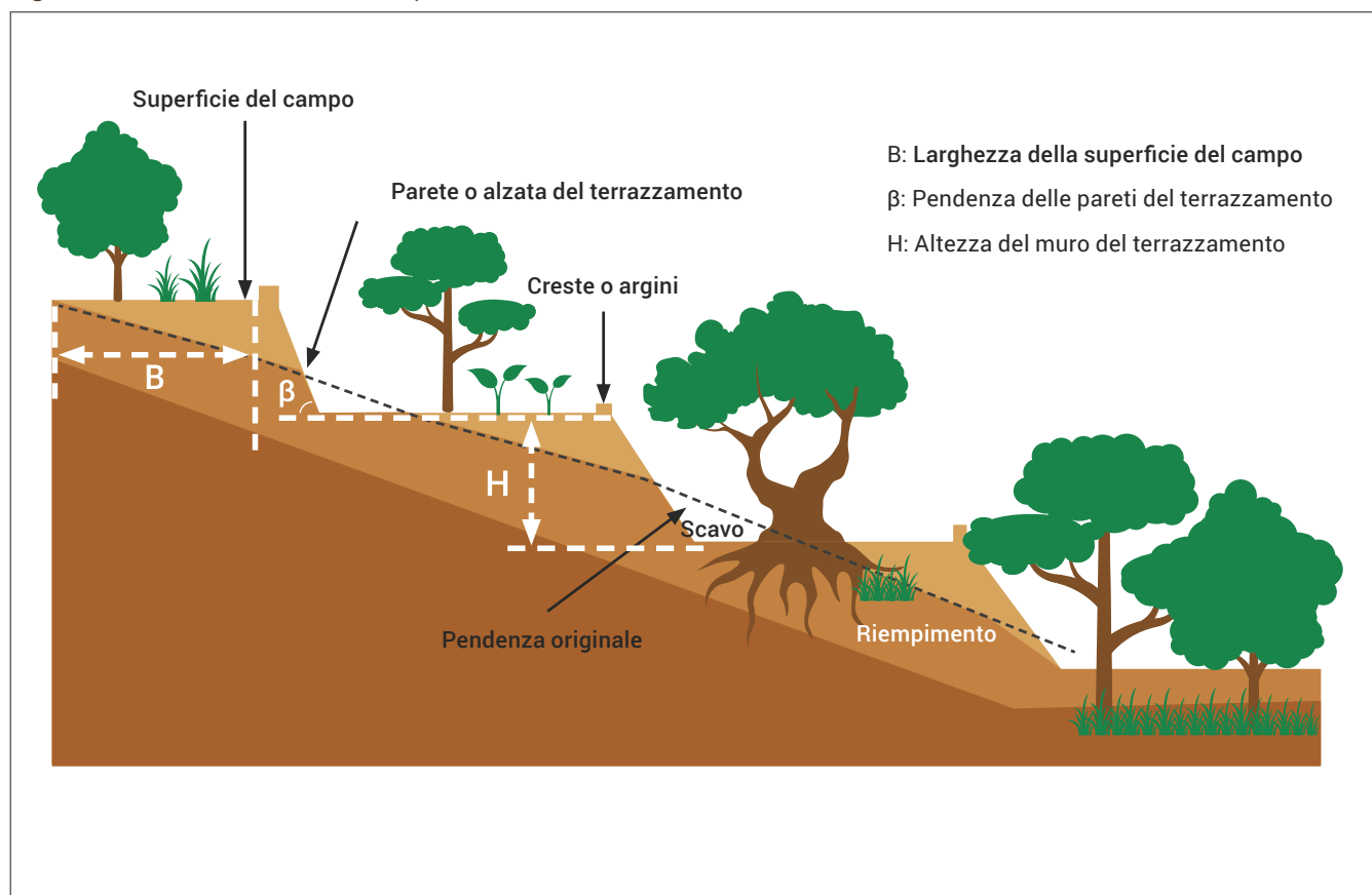
Figura 3.1 Schema in sezione di un pendio terrazzato
