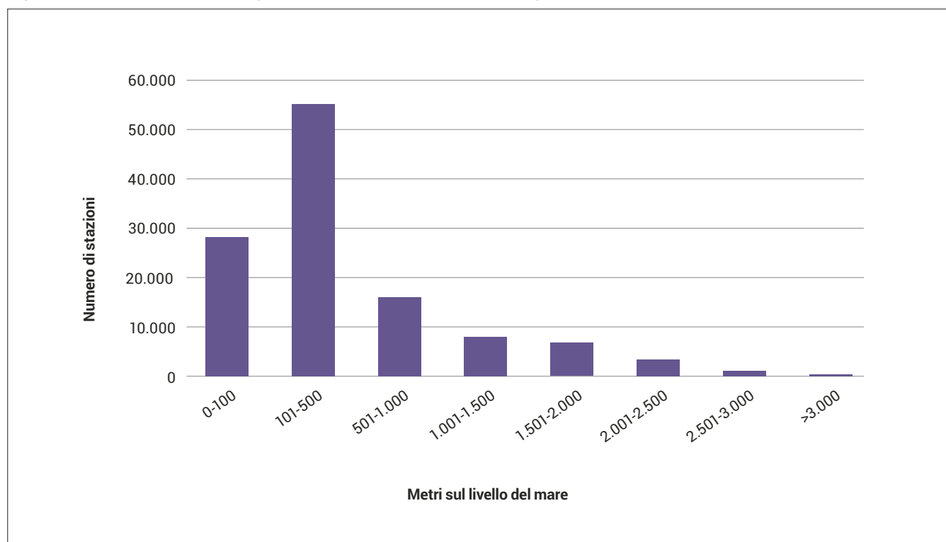
Figura 8.1 Distribuzione storica globale delle stazioni idrometeorologiche per altitudine, 1750-2024
