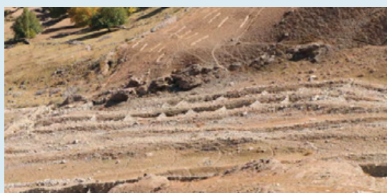
Barrages de retenue, digues de terre et plantations d'arbres visant à stabiliser les pentes
